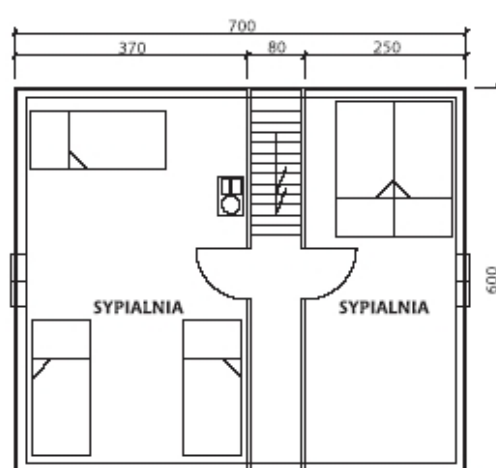
Rzut poddasza
