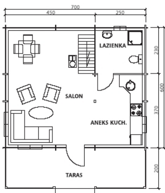
Rzut parteru
